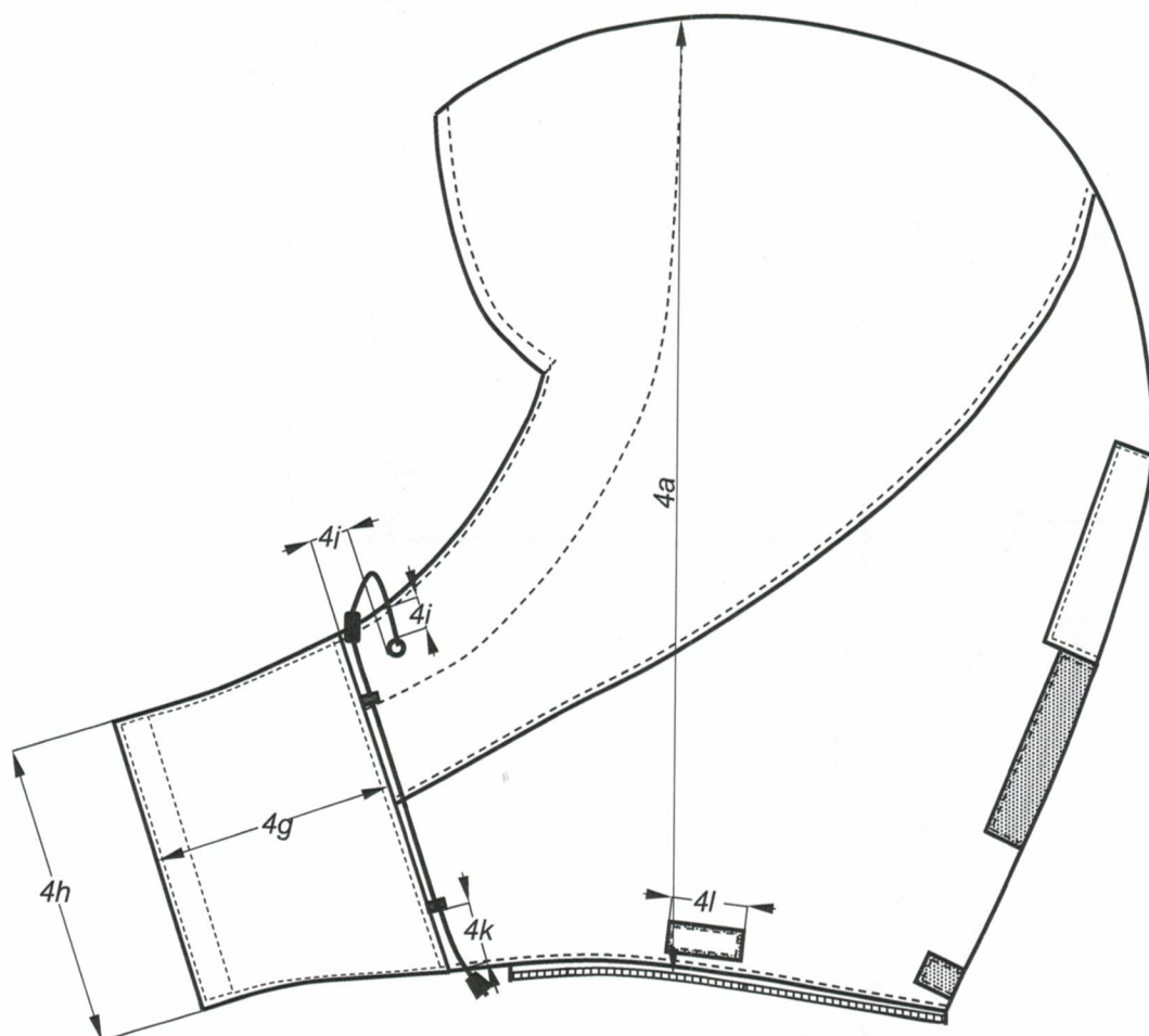
Rysunek 4 - Kurtka - góra tyłu
