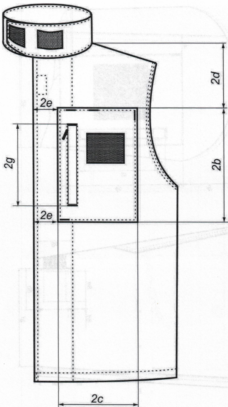
Rysunek 3 – Przód bluzy rozmieszczenie kieszeni
