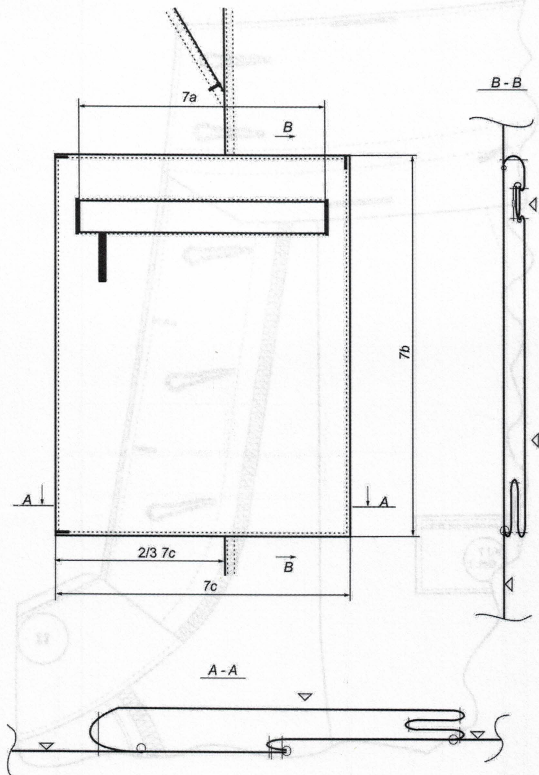
Rysunek 8 – Kieszeń udowa
