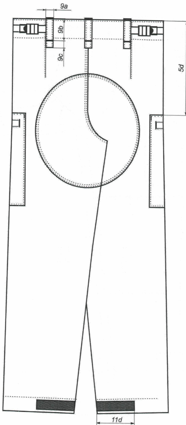
Rysunek 7 – Tył spodni
