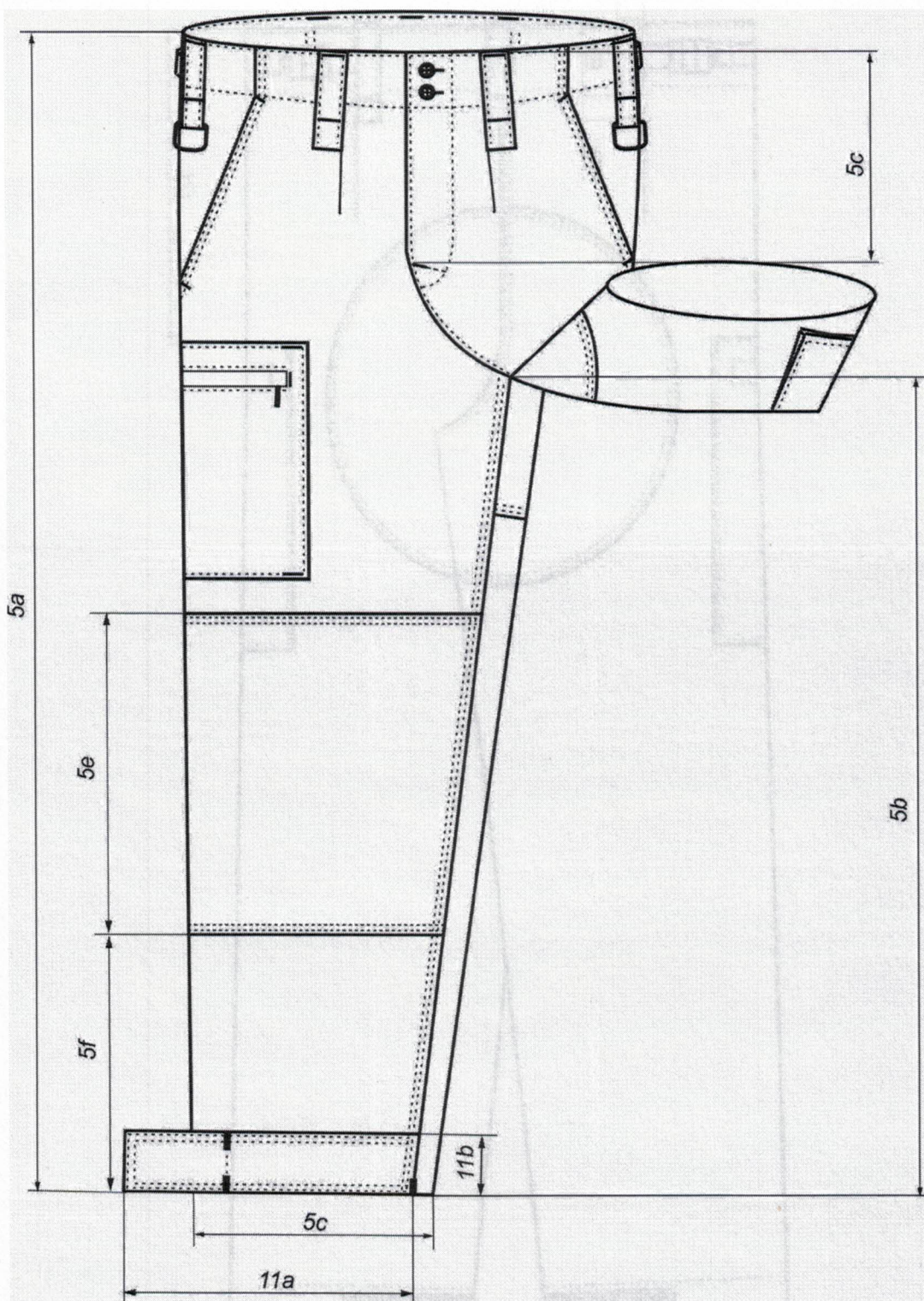
Rysunek 6 – Przód spodni
