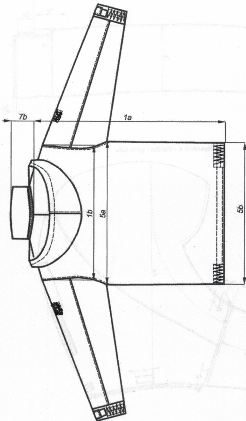
Rysunek 3 - Kurtka -tył
